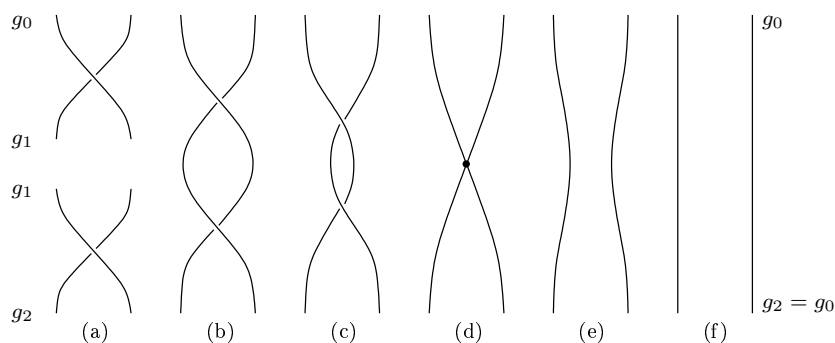
FIGURE 6.3 – Dégénérescence de tresses quantiques
