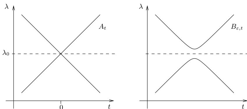
FIGURE 6.2 – Perturbation d'une valeur propre double
