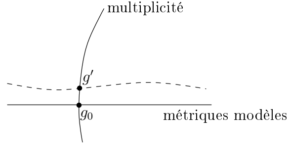
FIGURE 6.1 – Propriété de transversalité d'une valeur propre multiple
