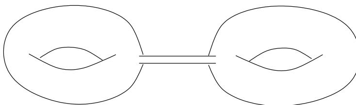
FIGURE 1.1 – Haltère de Cheeger
