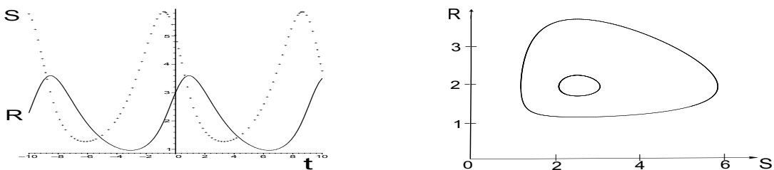
FIGURE 1 – A gauche le graphe des effectifs des proies S(t) (en pointillés) et celui des prédateurs R(t) (en trait plein), dans le cas où S(0) = 5 et R(0) = 3 . A droite plusieurs trajectoires du système (2) représentées dans le plan de phase (la trajectoire extérieure est issue du point de coordonnées (S(0) = 5 ; R(0) = 3) et correspond aux deux graphes de gauche).
